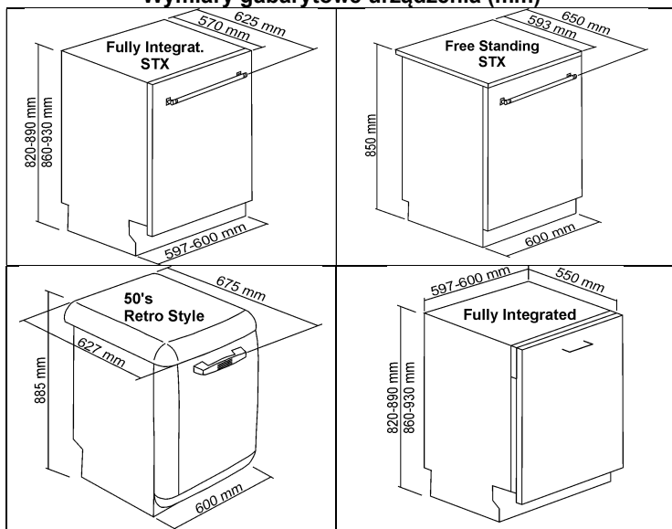
Wymiary gabarytowe urządzenia (mm)
