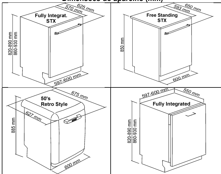
Dimensões do aparelho (mm)
