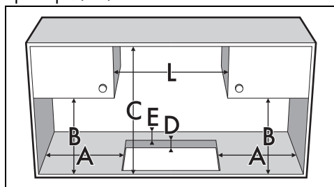
Размеры мебели для встраивания прибора (мм)
