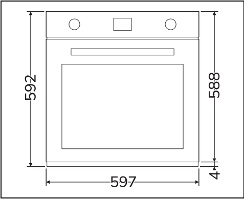
Габаритные размеры прибора (мм)
