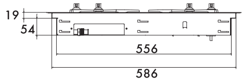
Vista traseira
