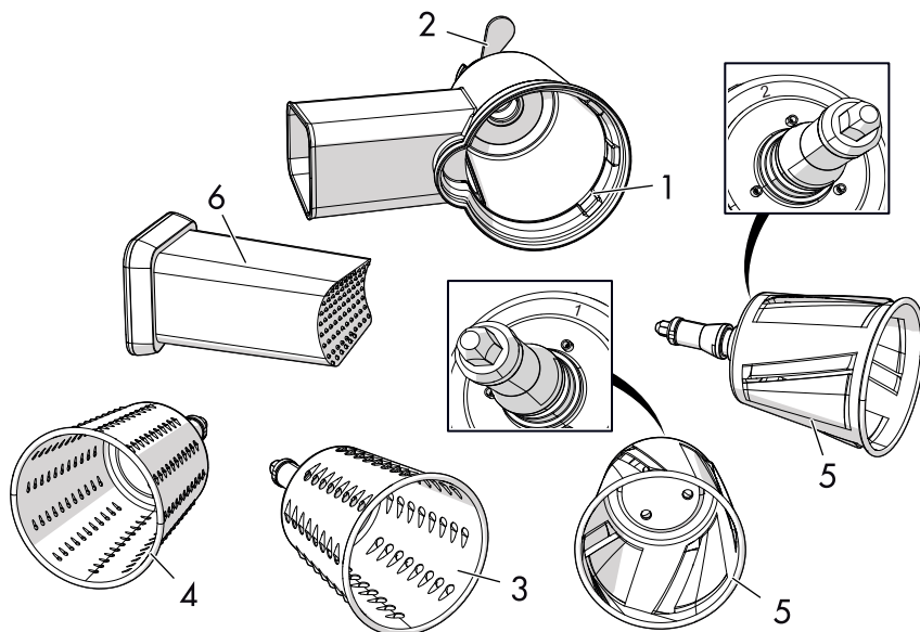
SMSG01 - Accesorio rallador de cilindros
