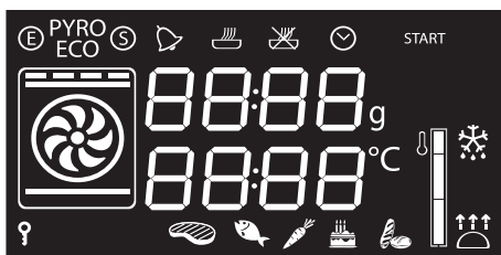
Pyrolysemodelle
